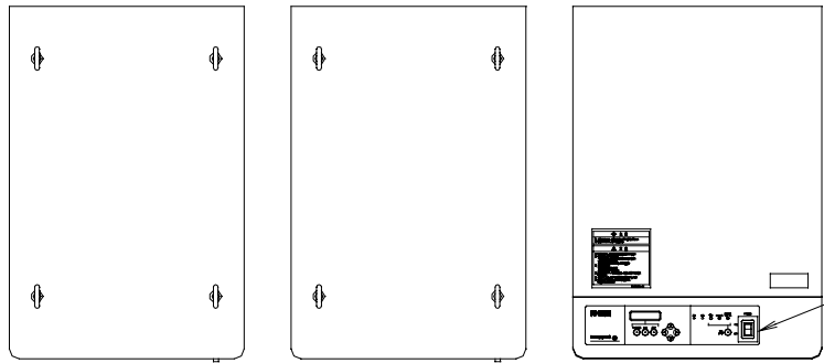
正面
