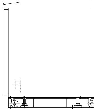
右側面
