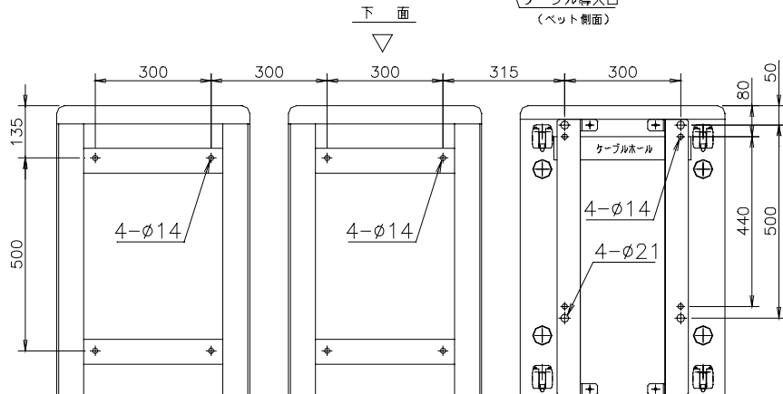
下面
