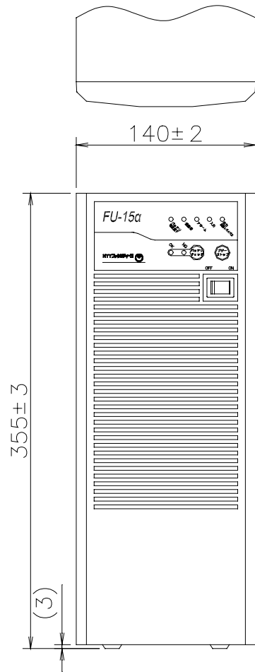
正面図
