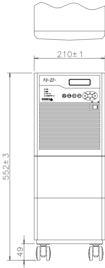
正面図
