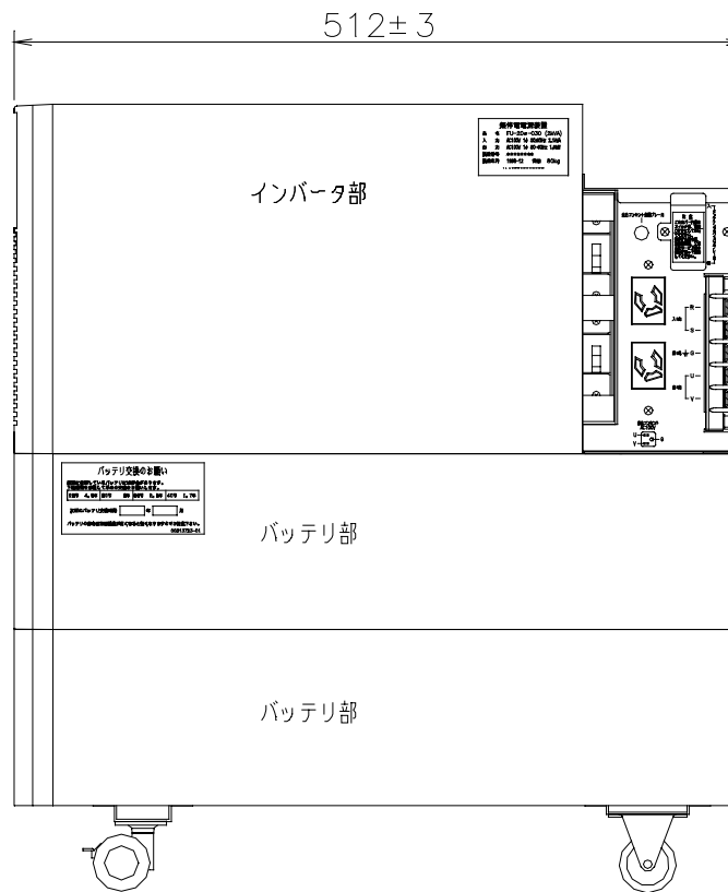
側面図
