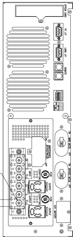
背面 入出力端子 及び操作スイッチ 詳細
