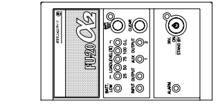
正面 表示及び操作部 詳細
