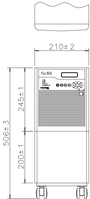
正面図
