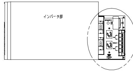
側面図 600±3
