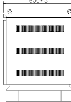
側面図 600±3
