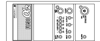
正面 表示及び操作部 詳細
