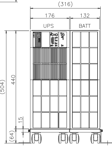
正面
