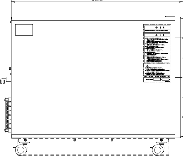
左側面
