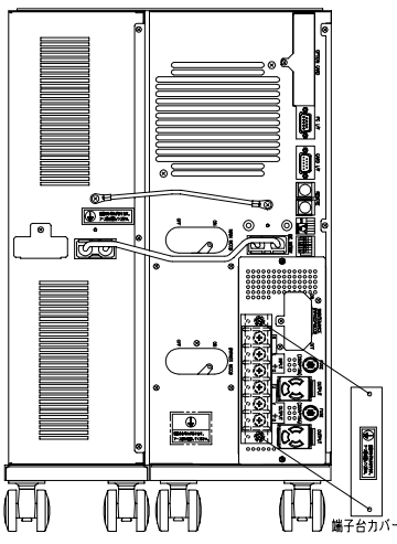
背面
