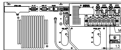
背面 入出力端子 及び操作スイッチ 詳細
