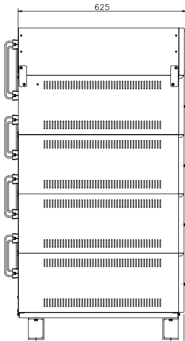
左側面
