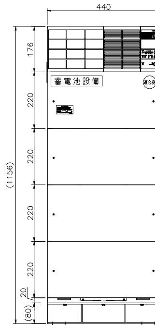
正面
