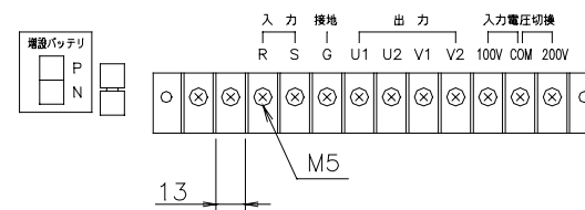
UPS入・出力端子台
