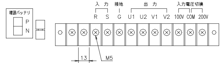
バッテリー盤 操作・接続部
