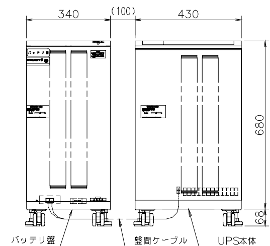
正面
