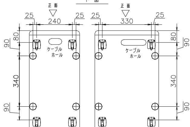
下面
