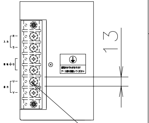
入出力端子
