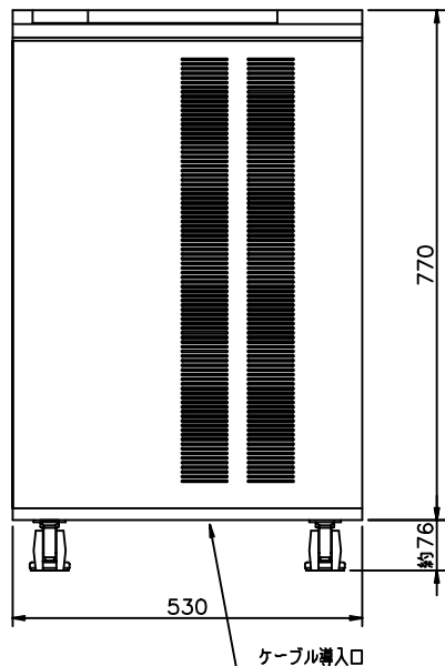
正面
