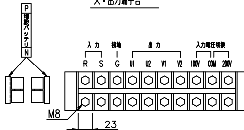
入・出力端子台
