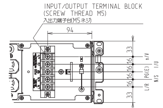
INSIDE VIEW OF TB COVER (REAR) TBカバー内部 (背面)
