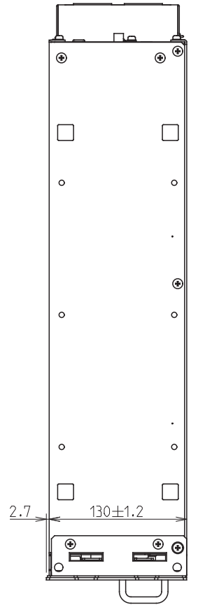
LEFT SIDE VIEW 左側面
