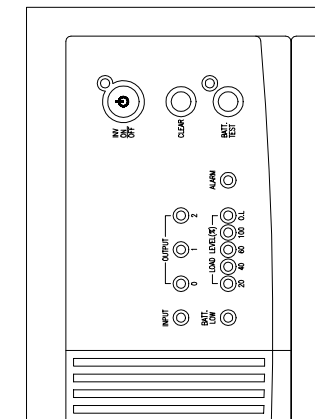
正面操作・表示部
