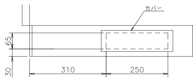
ケーブルホール詳細図
