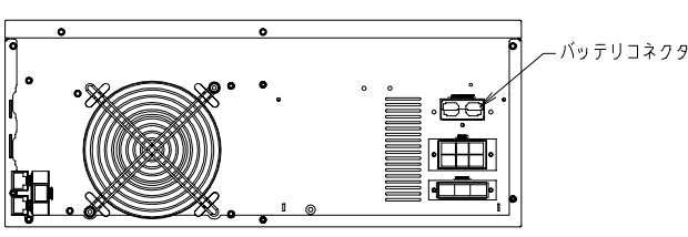
UPSユニット背面(ケーブルカバーなし)
