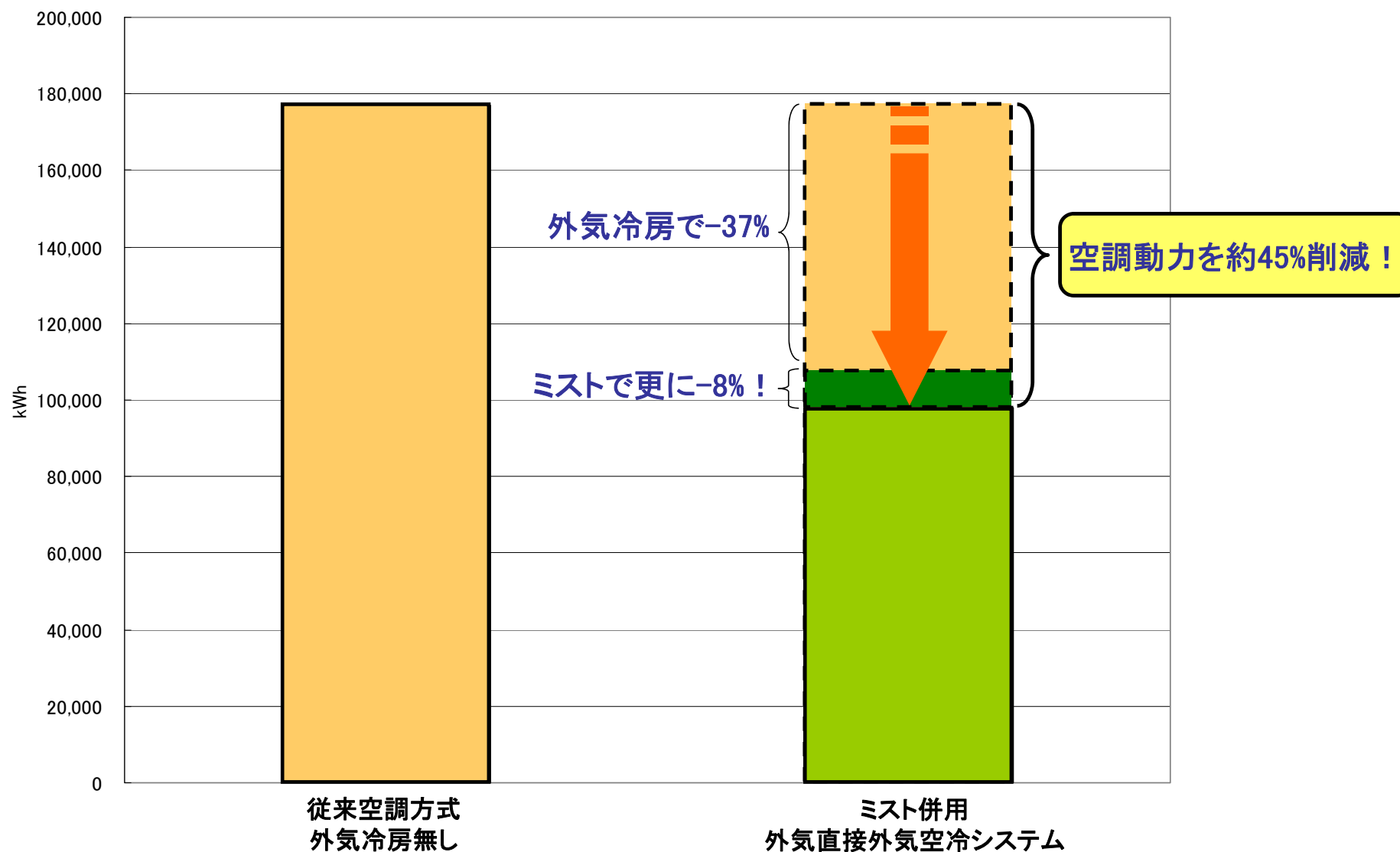
年間消費電力量比較
