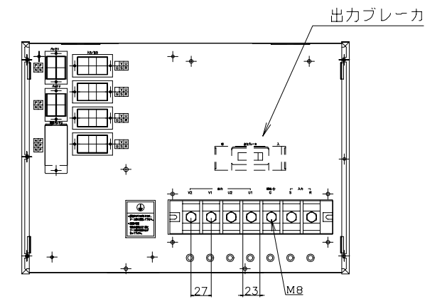
集電箱入出力部
