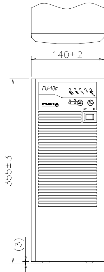
正面図
