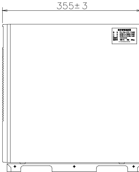
側面図
