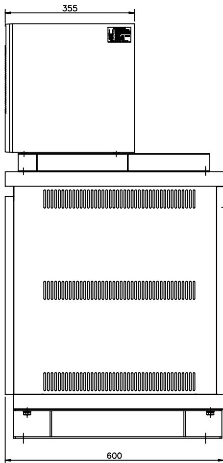
床固定寸法
