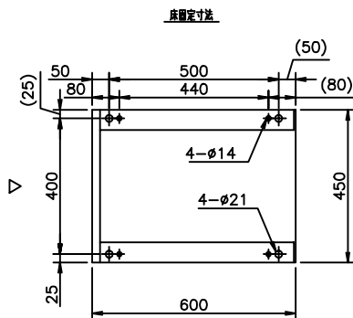
床固定寸法
