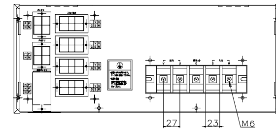
集電箱入出力部
