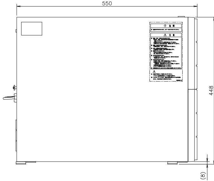
左側面
