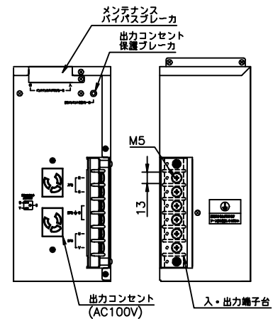
UPS 入・出力端子台
