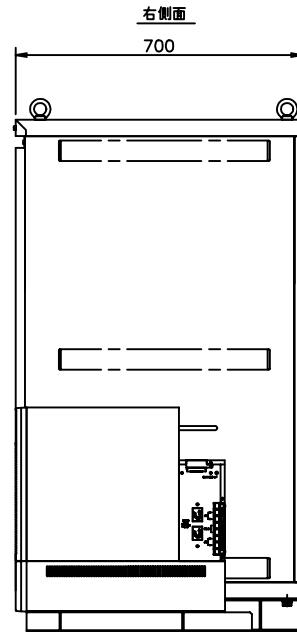
バッテリー盤 操作部
