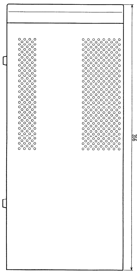
右側面図
