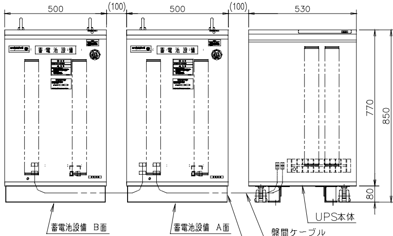
正面
