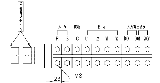
UPS本体 入・出力端子台部
