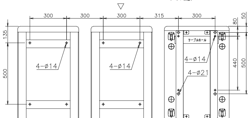
下面
