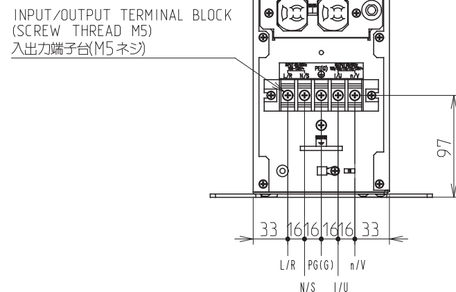
INSIDE VIEW OF TB COVER TBカバー内部
