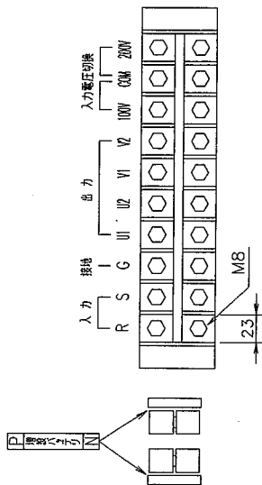
UPS本体 入・出力端子台
