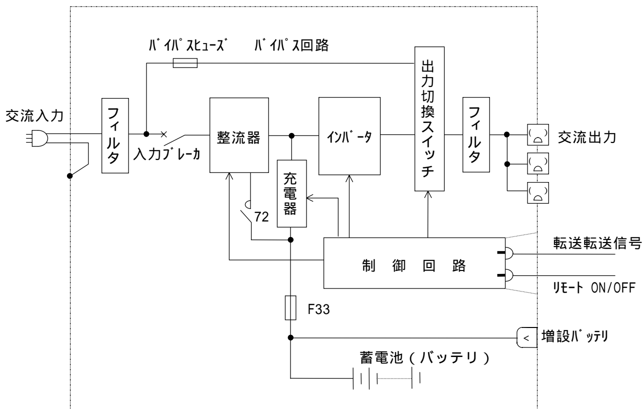
回路系統図
