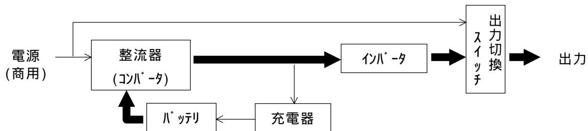
商用電源異常時の電力供給経路
