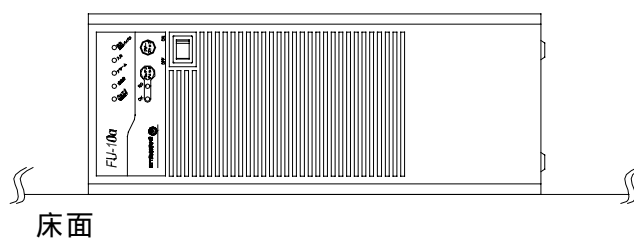
横置き設置例
