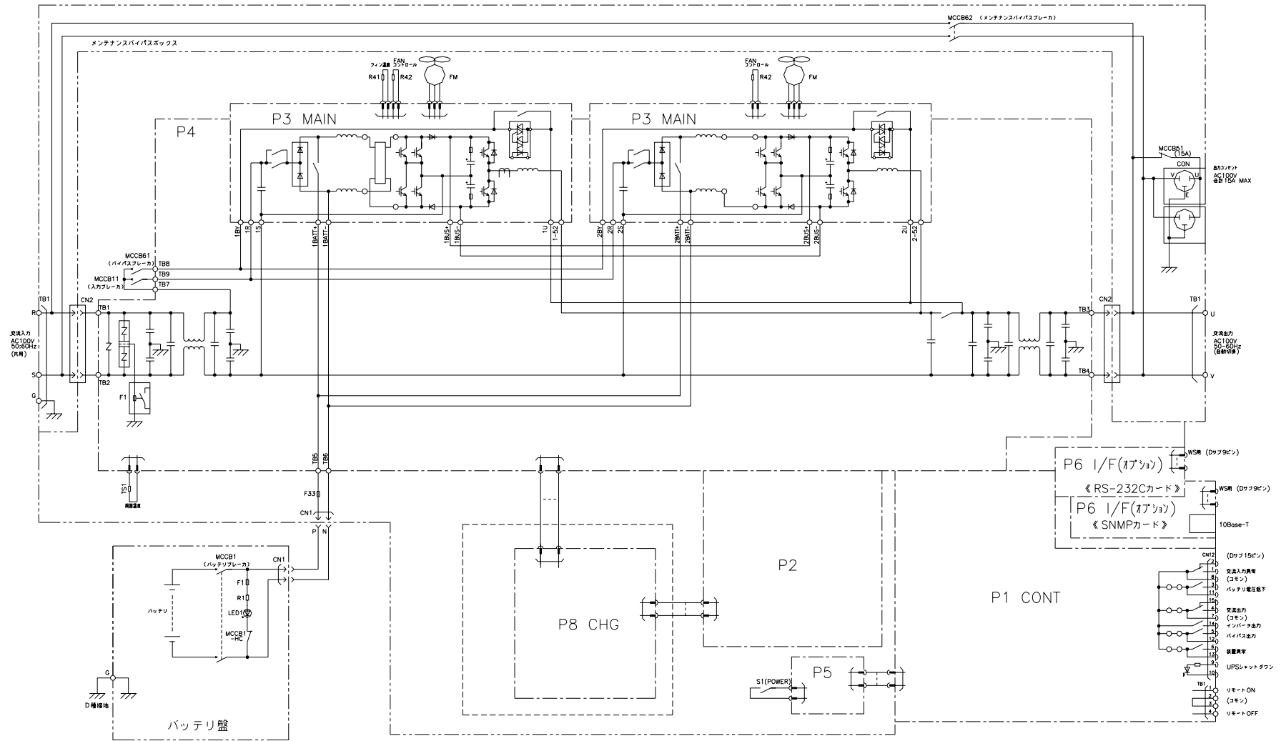
FU-20-030-L 電気回路図
