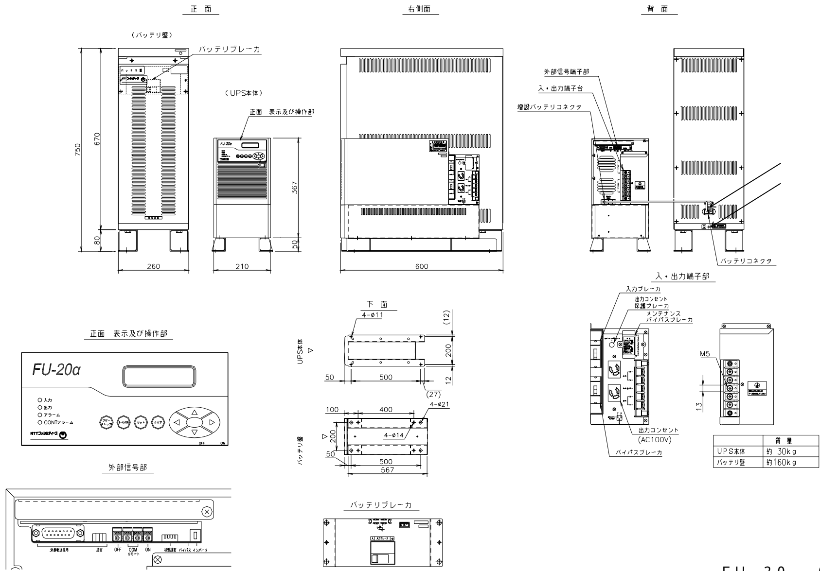
FU - 20 - 030 - L 外観構造図 (UPS本体 床置き)
