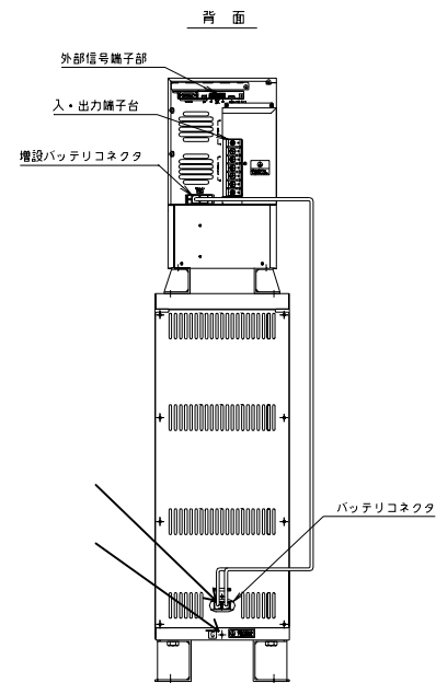
入・出力端子部
