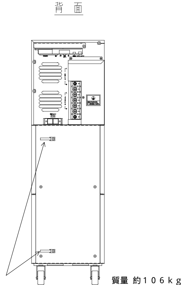
FU-30-030 外観構造図
