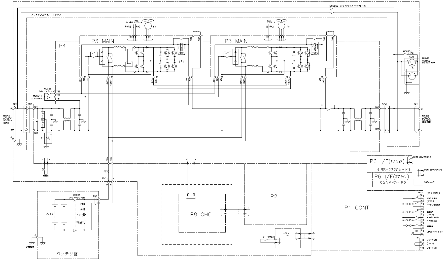
FU-30-060-L 電気回路図
