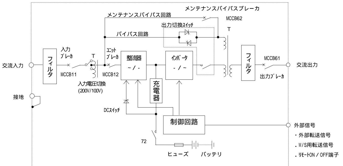
回路系統図
