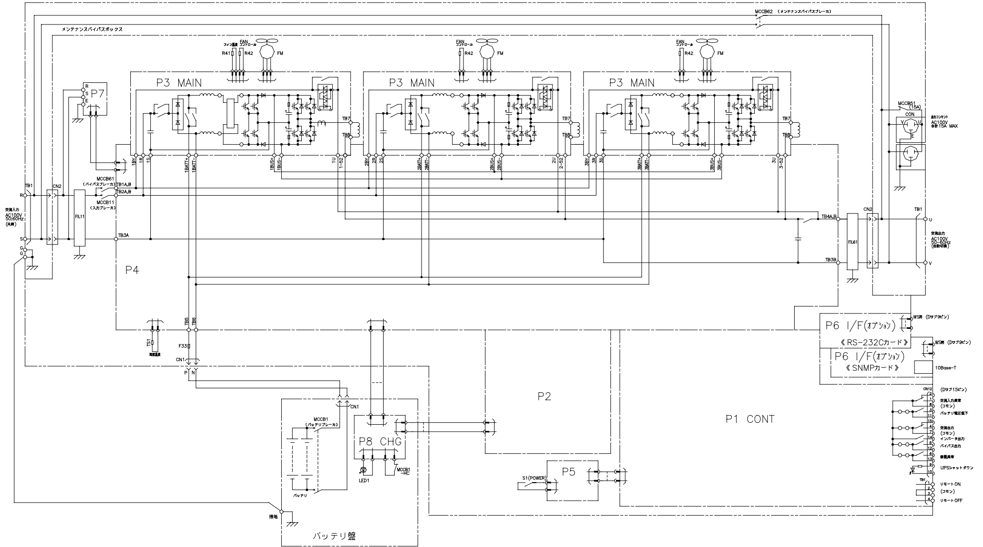
FU - 50 - 060 電気回路図
