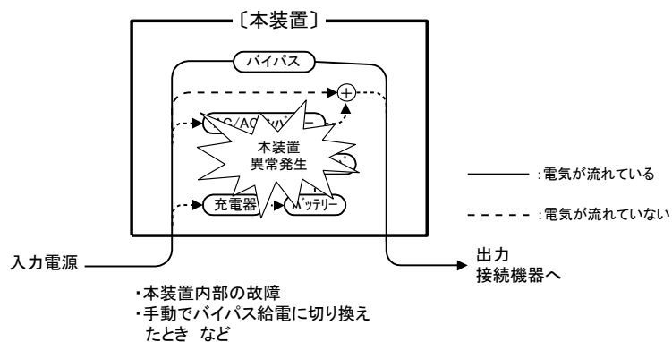
バイパス運転時の電気の流れ
