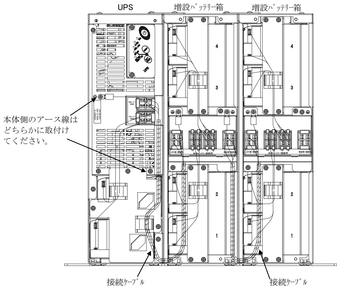
内部正面(増設バッテリー箱2台の時)
